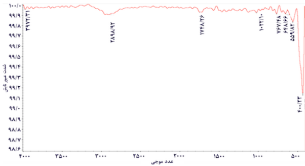
نمودار ۶ - آزمون FTIR برای پوشش نانو نقره
